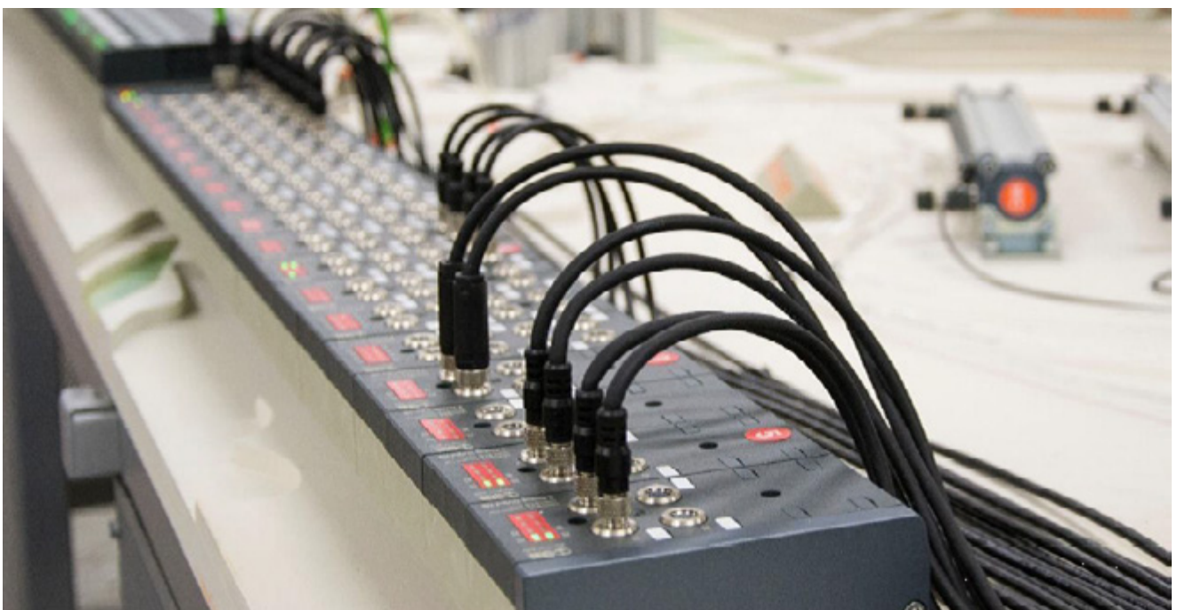
Figura 4: EB 80 gestisce attuatori e sensori, sia in analogico che in digitale.
