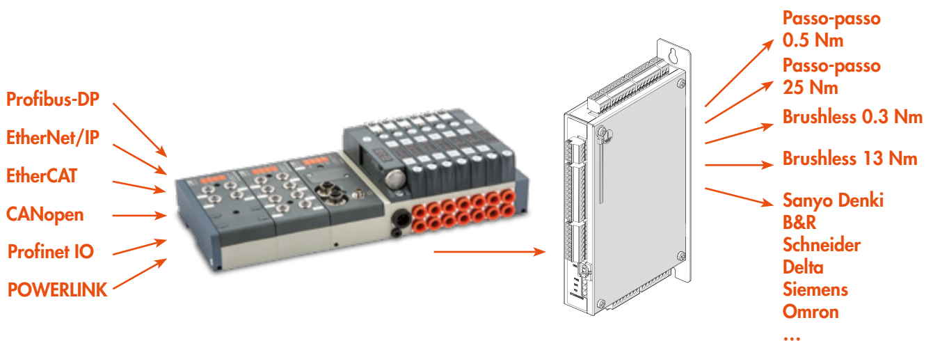
Figura 9: Il dispositivo E-motion permette di collegare qualsiasi tipo di bus di campo a qualsiasi marca e potenza di azionamento per motori passo-passo o brushless
