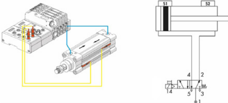
Figura 5: Il sistema gestisce anche i dati degli attuatori collegati, numero di cicli, velocità, ritardi, guasti.
